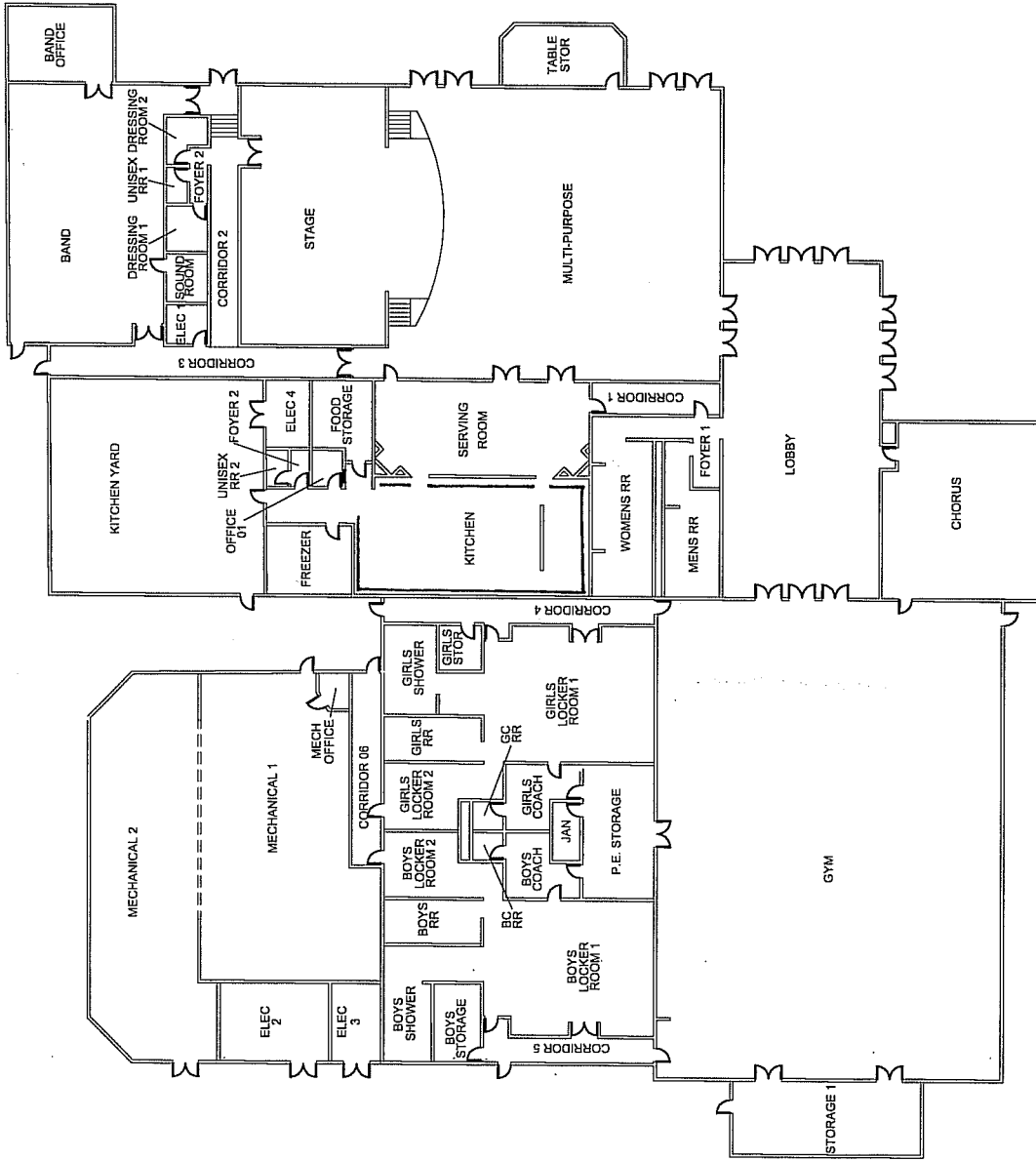
FLOOR PLAN N.T.S.
