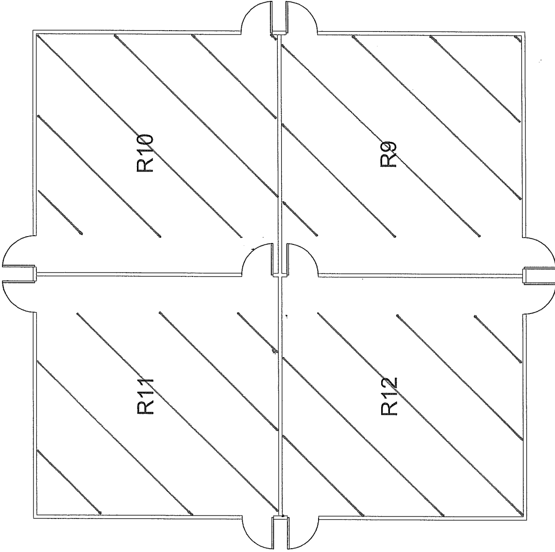
FLOOR PLAN N.T.S.
